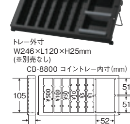
フタの開閉に連動してコイントレーが立ち上がります。
